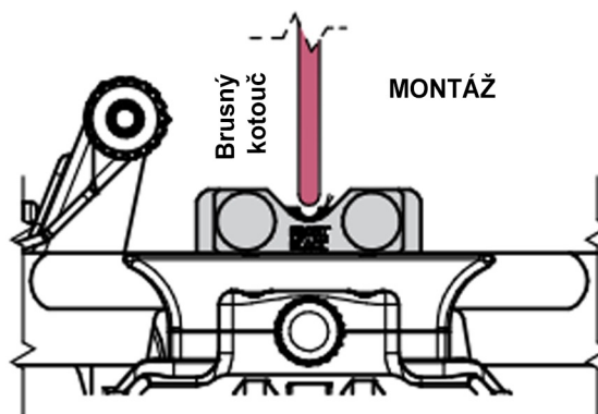
Přední pohled v upínacím zařízení
